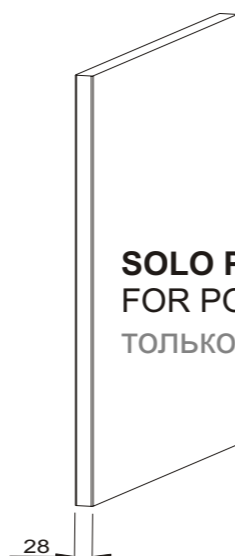
FIANCO A FINIRE END PANEL отделочная панель 2430/870 x 580 x 28 960 x 335 x 28
