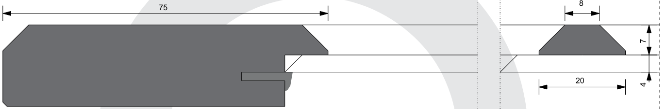
przekrój WS1_szkło / section WS1_glass
